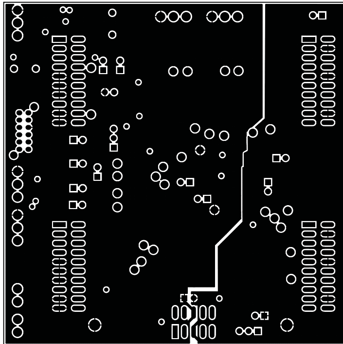
Figure C-3. Layer 3
